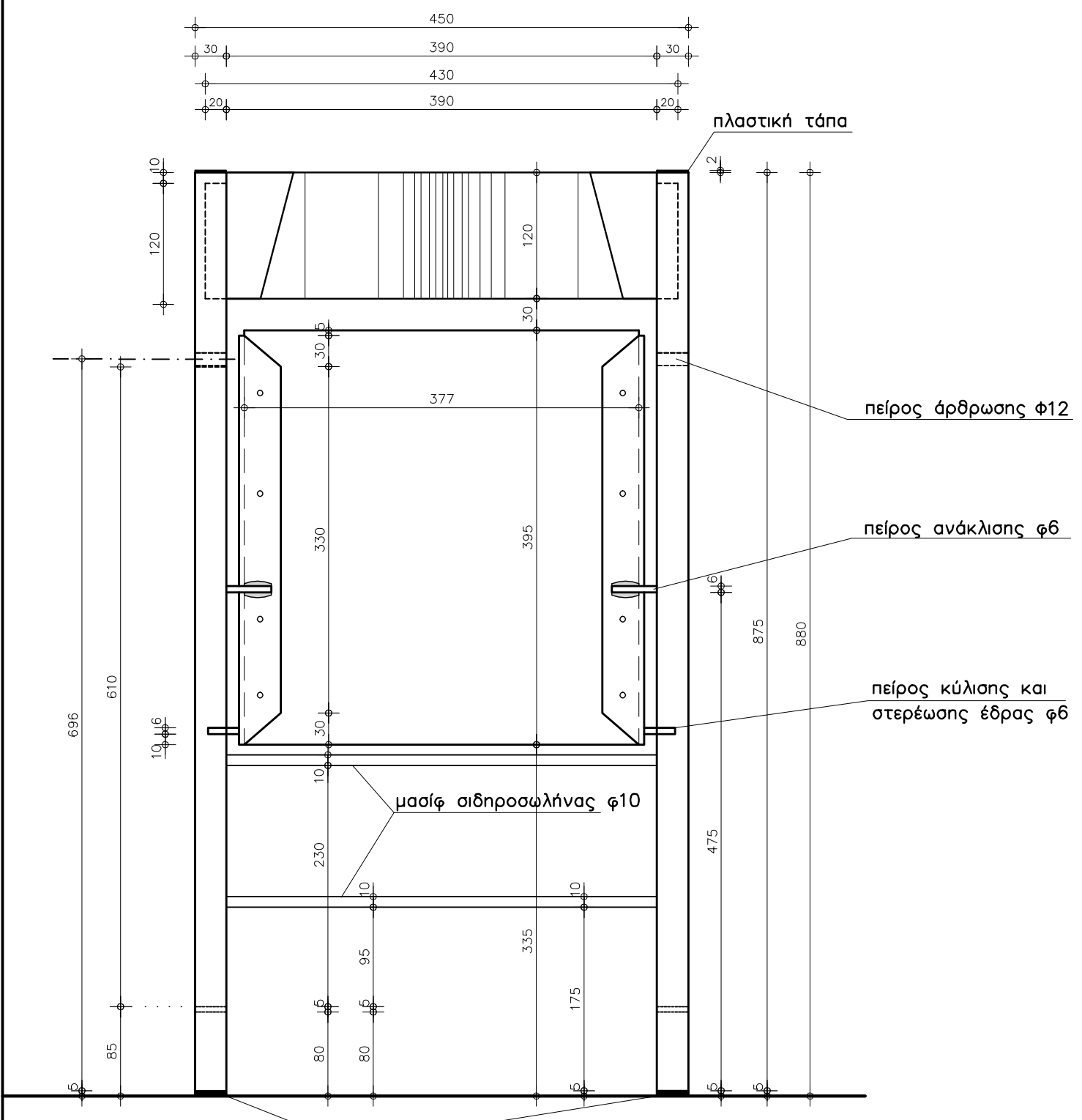
ΟΨΗ ΚΑΘΙΣΜΑΤΟΣ (ΚΛΕΙΣΤΗ ΘΕΣΗ)
