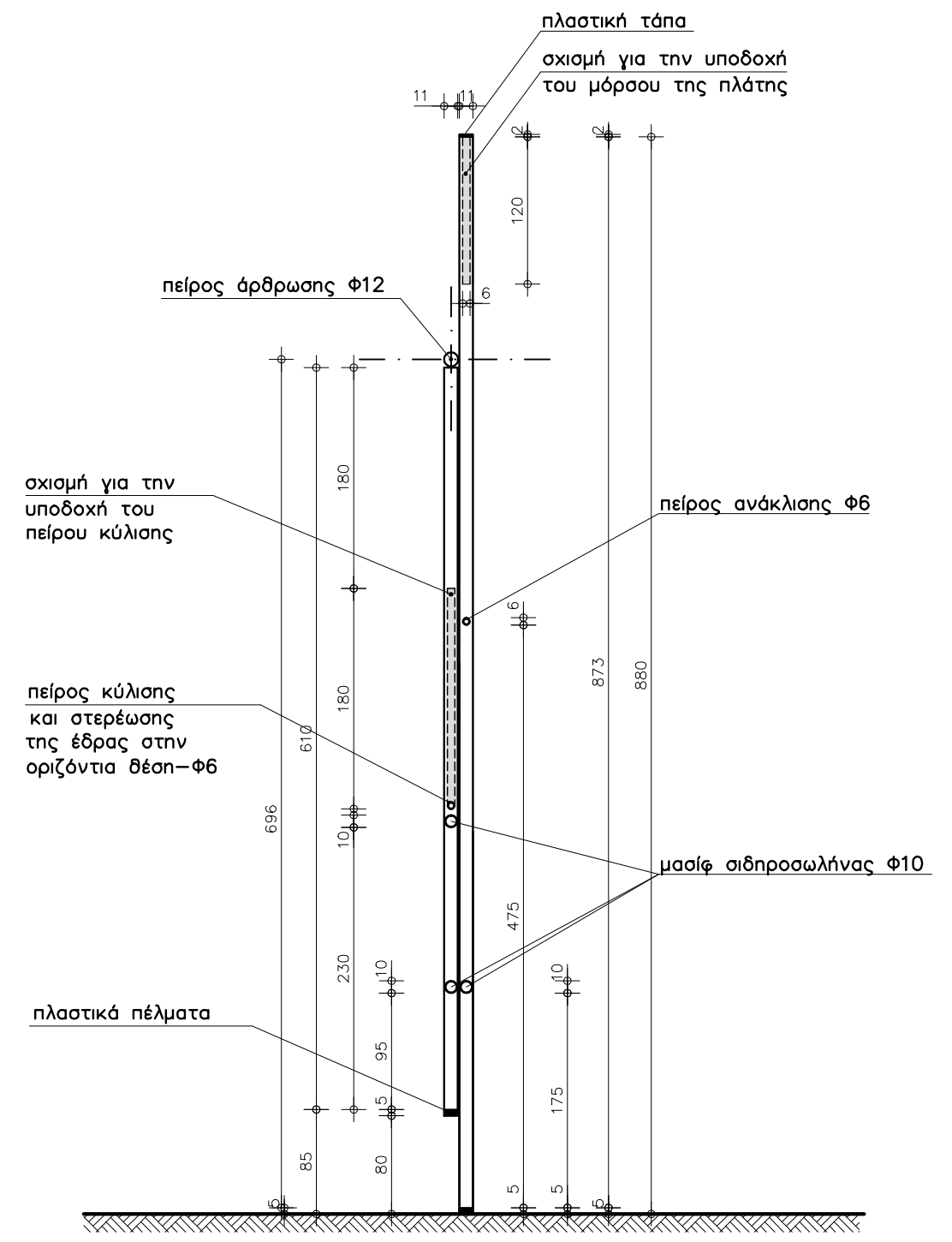
ΠΛΑΓΙΑ ΟΨΗ ΜΕΤΑΛΛΙΚΟΥ ΣΚΕΛΕΤΟΥ (ΚΛΕΙΣΤΗ ΘΕΣΗ)
