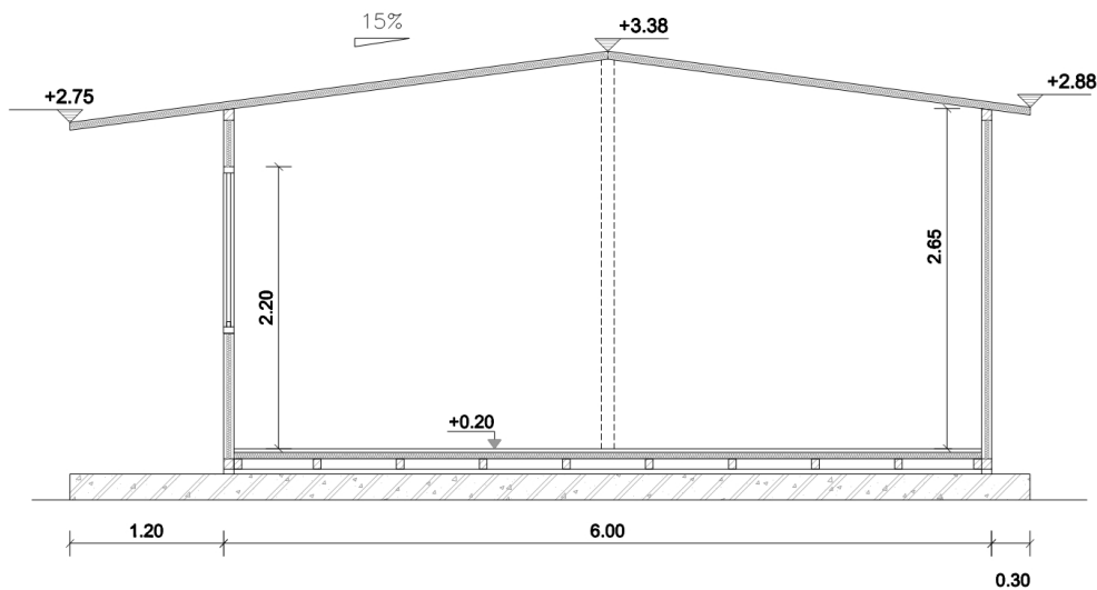
ΤΟΜΗ Τ2-Τ2
