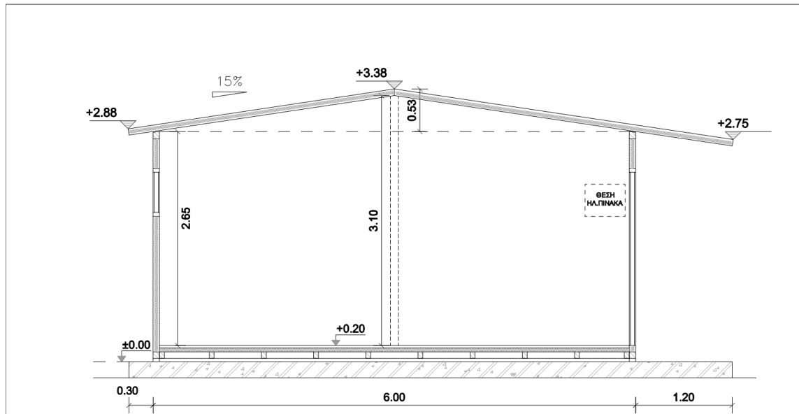
ΤΟΜΗ Τ1-Τ1
