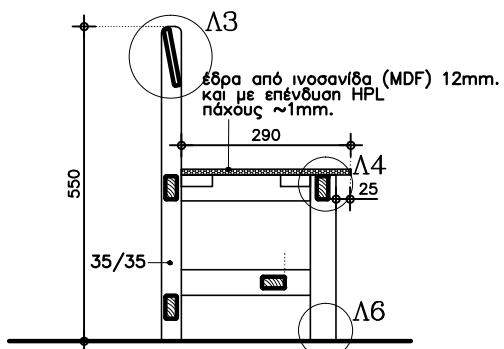
ΤΟΜΗ Τ1-Τ1 1:10
