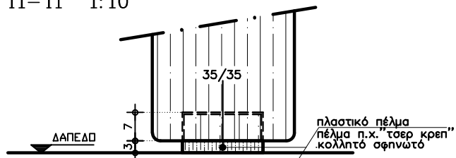
ΟΨΗ ΠΟΔΙΟΥ
