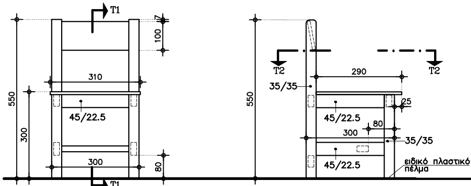
ΠΡΟΣΟΦΗ 1:10
