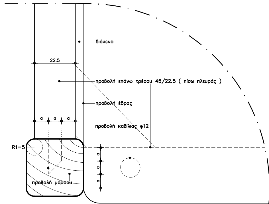
ΛΕΠΤΟΜΕΡΕΙΑ Λ1 1:1
