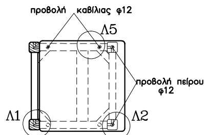
ΤΟΜΗ Τ2-Τ2 1:10
