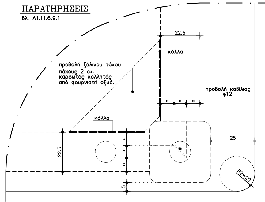
ΛΕΠΤΟΜΕΡΕΙΑ Λ2 1:1
