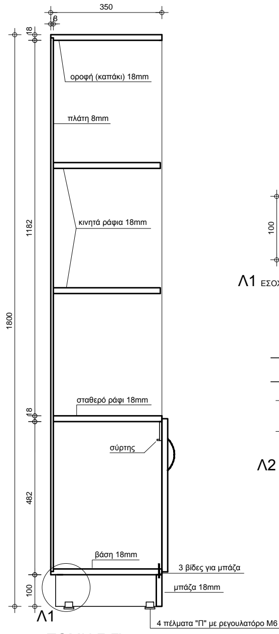
ΤΟΜΗ Γ-Γ'
