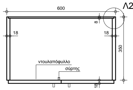
ΤΟΜΗ Β-Β'
