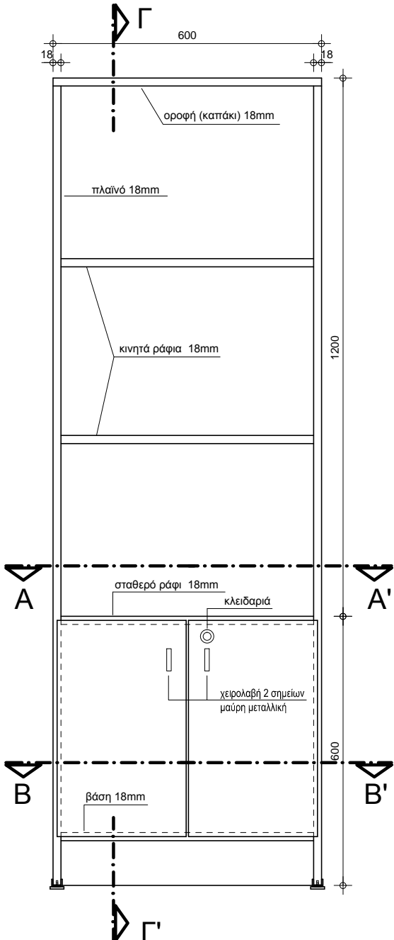
ΟΨΗ ΒΙΒΛΙΟΘΗΚΗΣ
